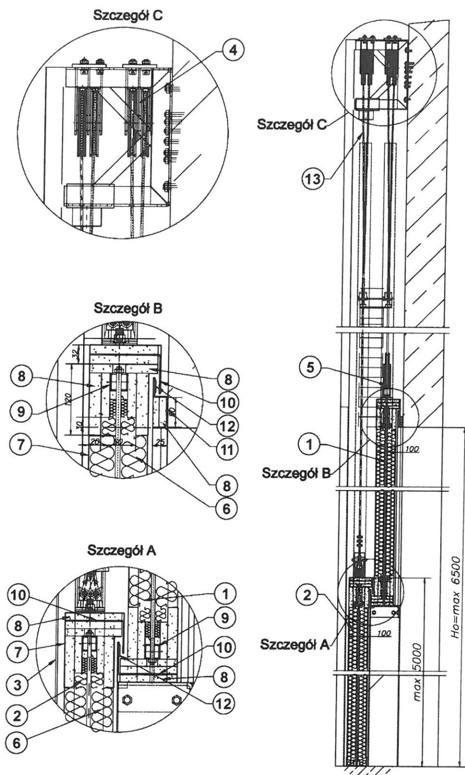
Rys. 30. Brama opuszczana MARC-Ot EI120. Przekrój pionowy
