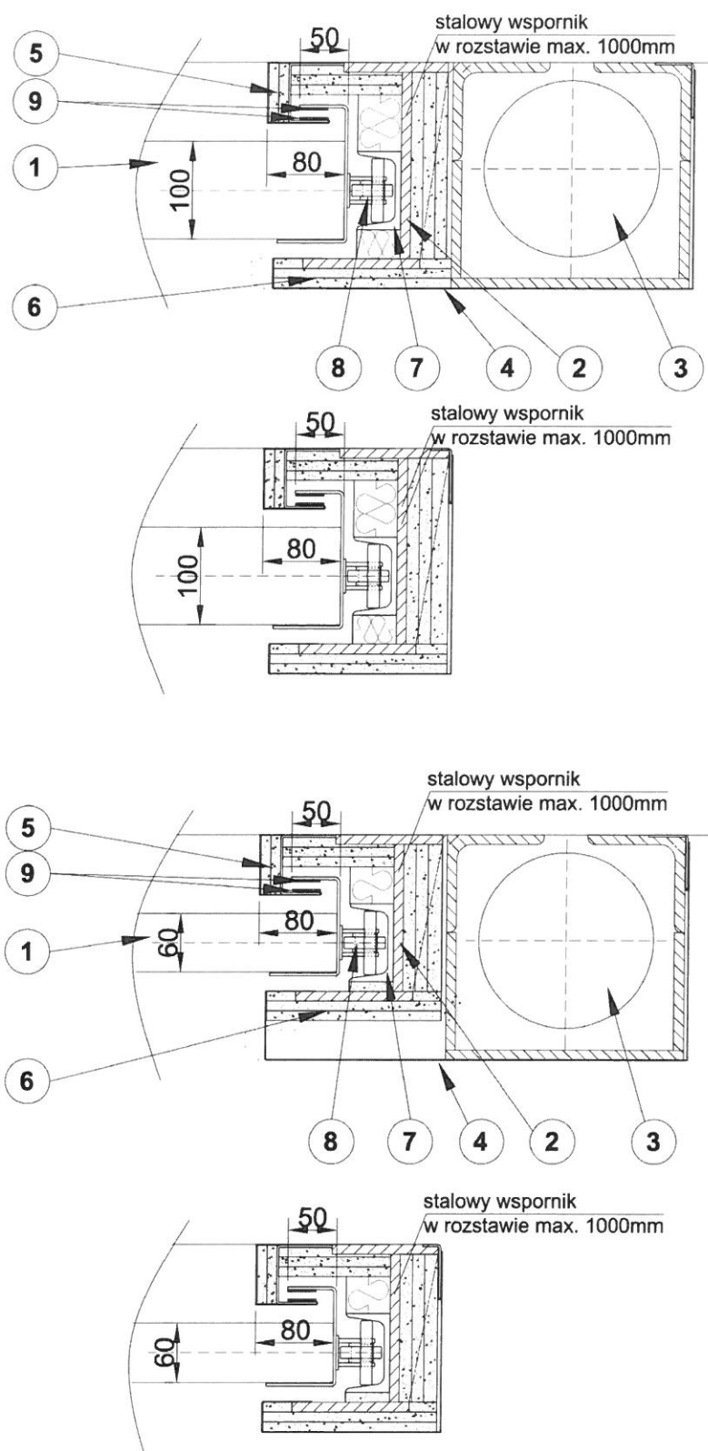
Rys. 36. Prowadzenie za pomocą prowadników łożyskowych bramy opuszczanej MARC-O
