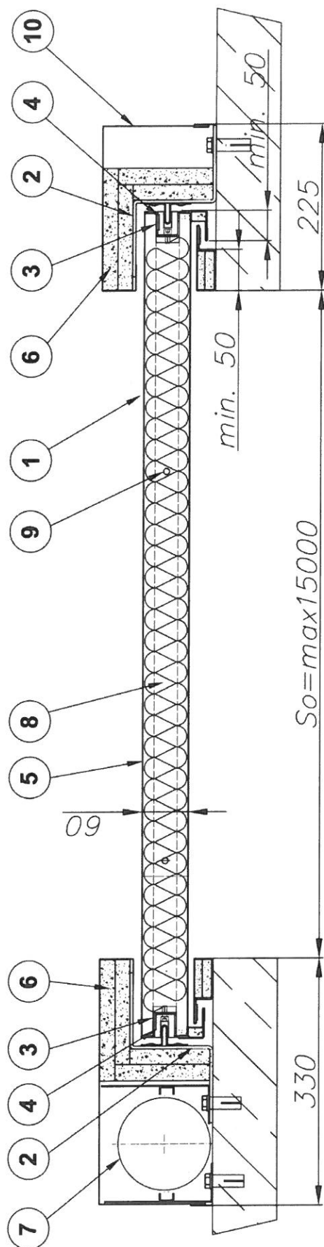
Rys. 28. Brama opuszczana MARC-O EI120. Przekrój poziomy
