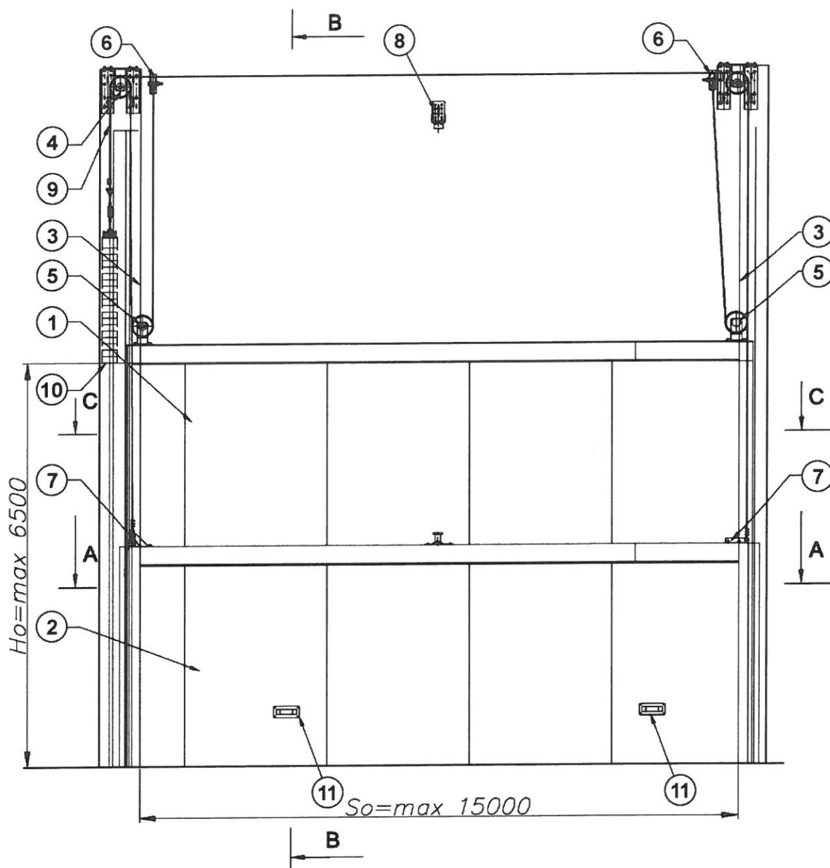
Rys. 29. Brama opuszczana MARC-Ot EI60. Widok
