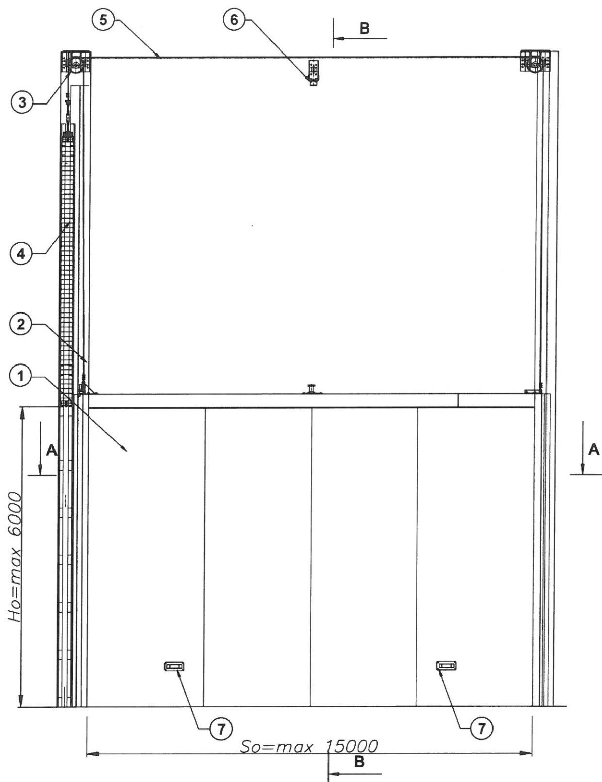
Rys. 23. Brama opuszczana MARC-O EI120. Widok
